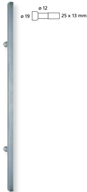
Stoßgriffe SG 16 \varnothing 25/13 Edelstahl matt
