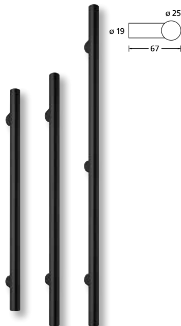
Stoßgriffe SG 16 \varnothing 25/19 Edelstahl schwarz
